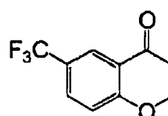
(I-38)
