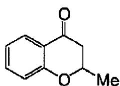
(I-46)
