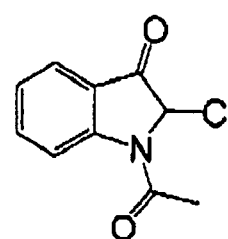
(I-127)
