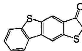
(I-85)
