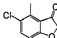
(I-91)
