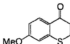
(I-10)
