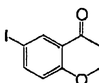
(I-37)
