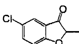
(I-96)
