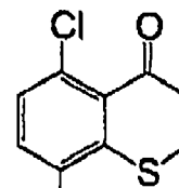
(I-9)
