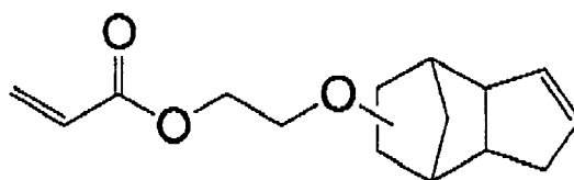
(FA-512A)
