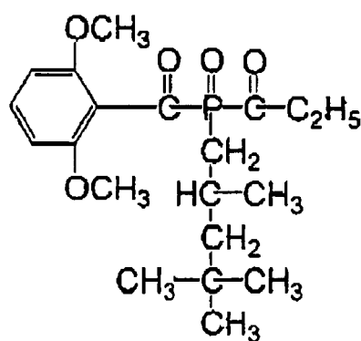
(P-23)
