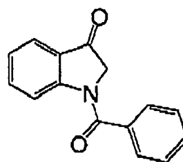
(I-124)
