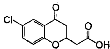
(I-52)
