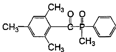
(P-17)
