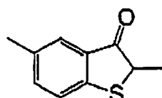
(I-75)
