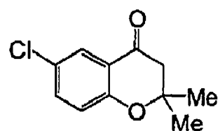
(I-50)
