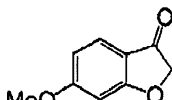
(I-93)
