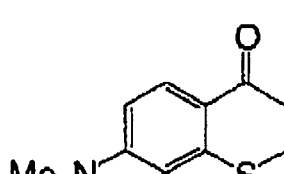
(I-11)
