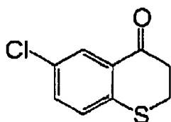
(I-4)
