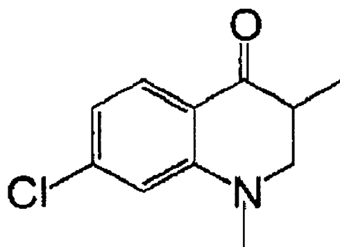
(I-116)
