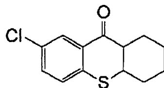
(I-130)
