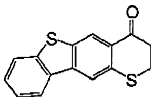
(I-28)
