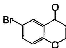
(I-36)
