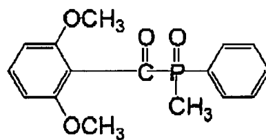
(P-18)
