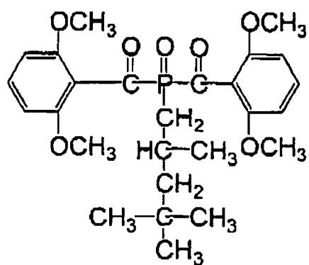
(P-22)
