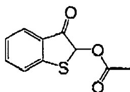
(I-80)
