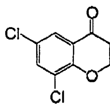
(I-39)
