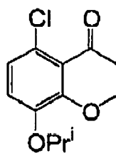
(I-40)
