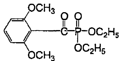
(P-14)
