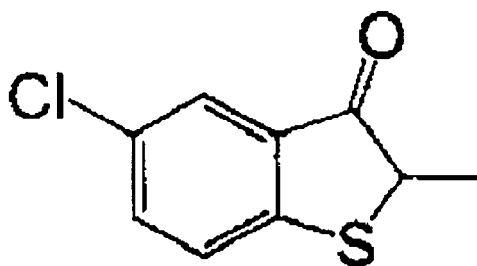
(I-71)
