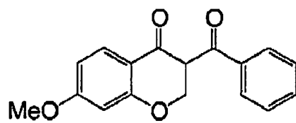
(I-51)
