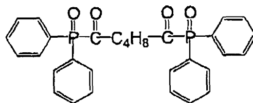
(P-10)
