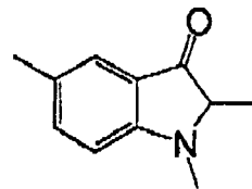
(I-121)
