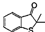
(I-76)
