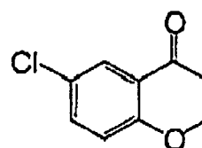
(I-35)
