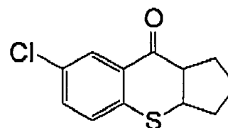
(I-131)
