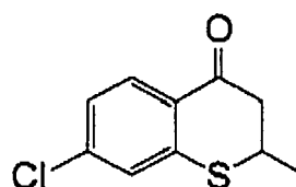
(I-129)
