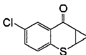
(I-133)
