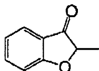
(I-98)
