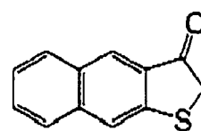
(I-82)
