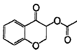
(I-54)
