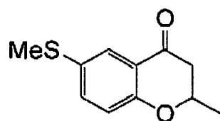
(I-128)
