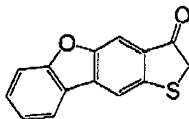
(I-87)
