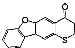
(I-30)
