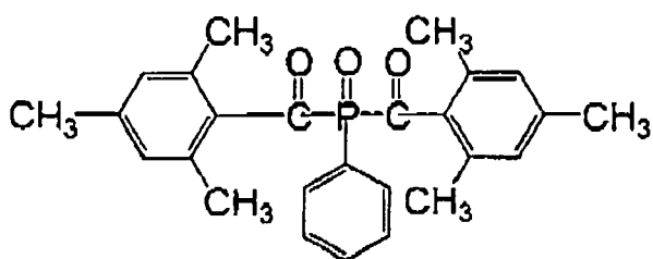
(P-19)
