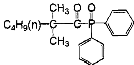
(P-7)
