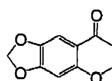
(I-58)
