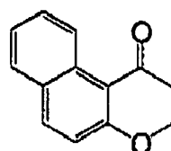
(I-57)
