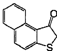
(I-83)
