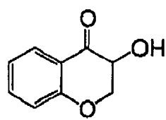
(I-53)
