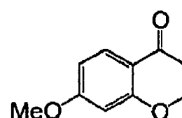
(I-41)
