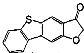
(I-110)
