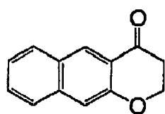
(I-56)
