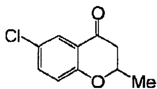
(I-45)
