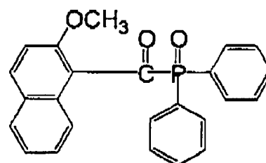
(P-16)
