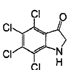
(I-122)
