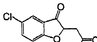
(I-103)
