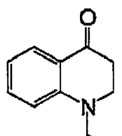
(I-117)
