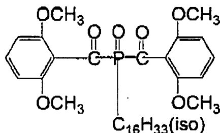
(P-25)
