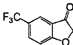
(I-90)
