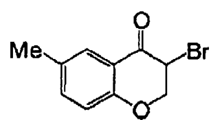
(I-44)
