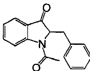
(I-126)
