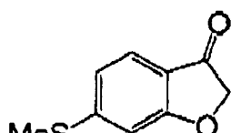
(I-95)
