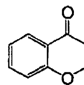
(I-32)
