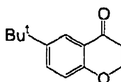
(I-34)
