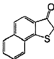
(I-81)
