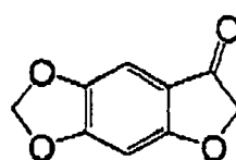
(I-111)
