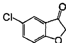
(I-89)
