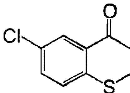
(I-4)
