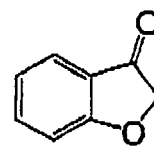
(I-88)
