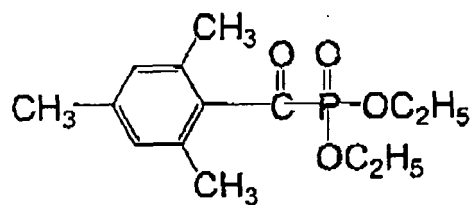
(P-5)
