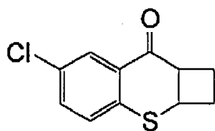
(I-132)
