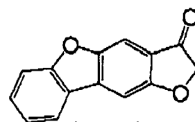
(I-112)
