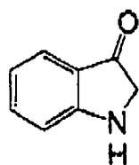
(I-119)
