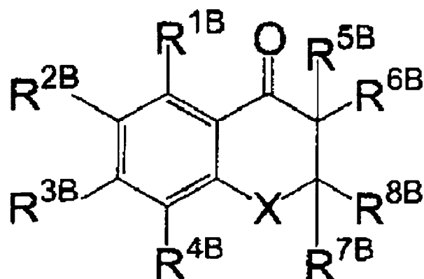
Formula (I-B)
