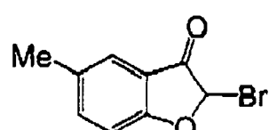
(I-97)
