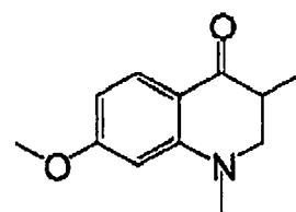
(I-118)
