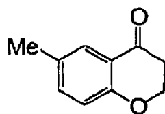
(I-33)
