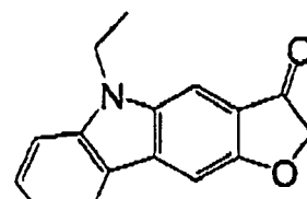
(I-109)
