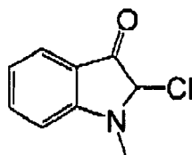
(I-120)
