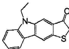
(I-84)
