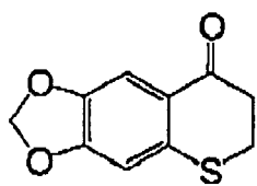
(I-27)
