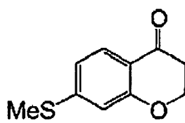
(I-43)
