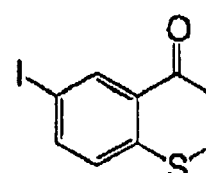
(I-6)
