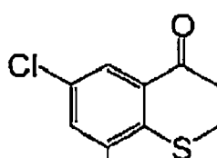
(I-8)
