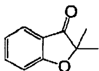
(I-101)
