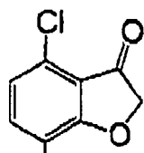
(I-92)
