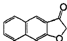
(I-107)
