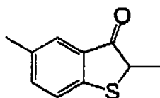
(I-74)
