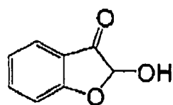
(I-104)
