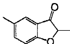
(I-99)
