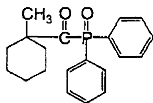
(P-11)
