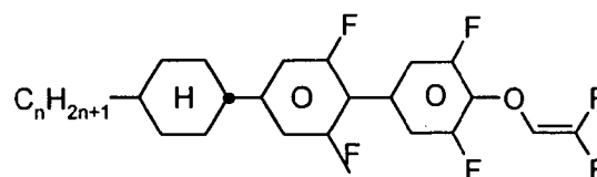
CUU-n-OXF
