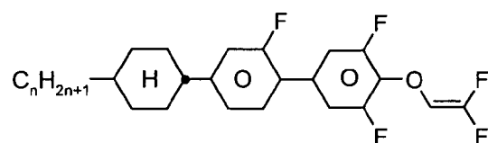
CCGU-n-F
