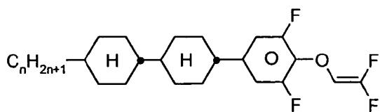
CCU-n-OXF
