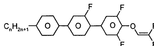
PGU-n-OXF
