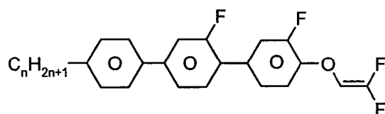
PGG-n-OXF
