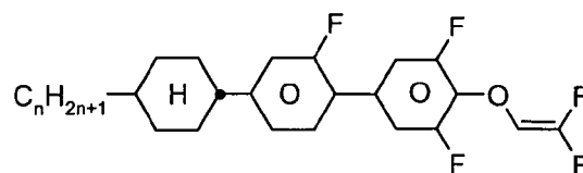
CGU-n-F
