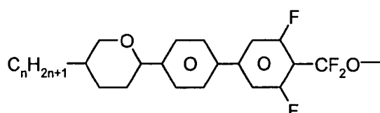
APUQU-n-F
