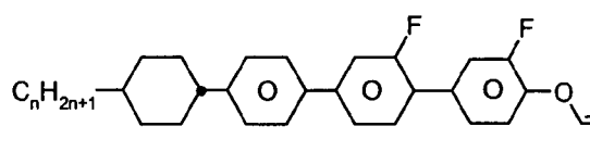
CPGU-n-OXF
