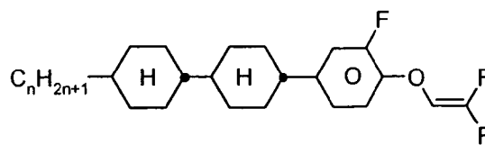
CCG-n-OXF
