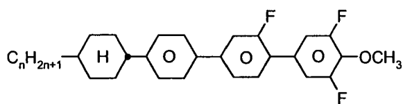
CPGU-n-OT
