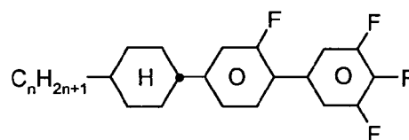
CGU-n-F
