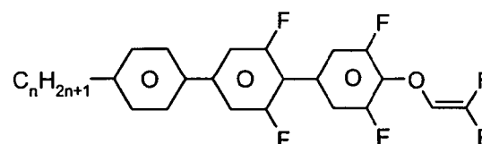
PUU-n-OXF
