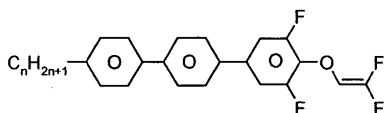
PPU-n-OXF
