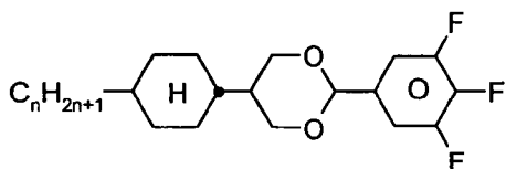
CDU-n-F
