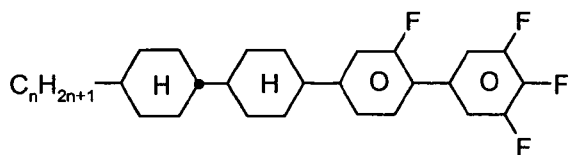
CCGU-n-F
