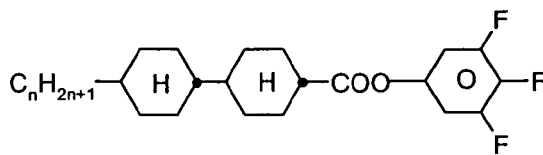
CCZU-n-F
