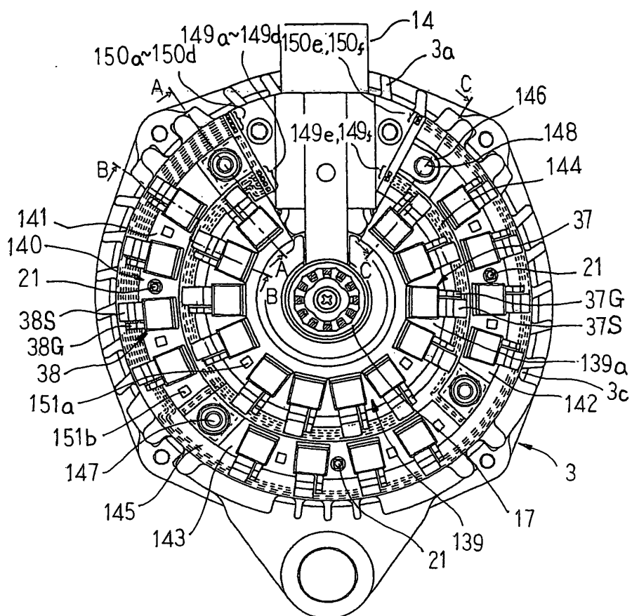
FIG. 24
