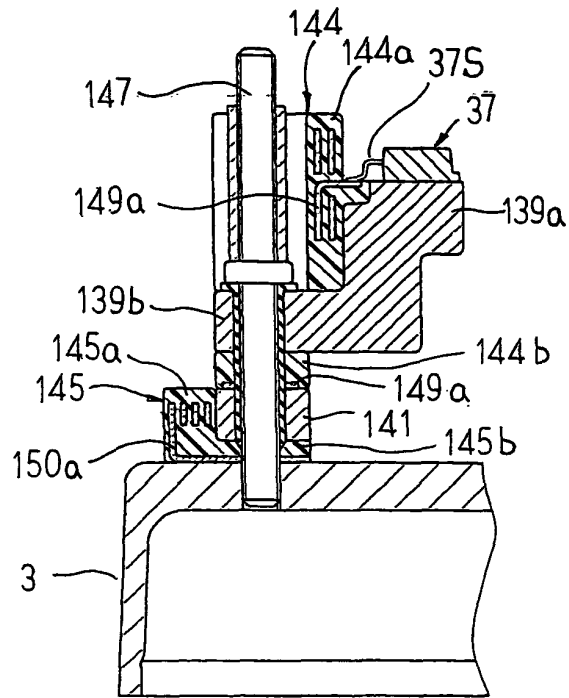
FIG. 25
