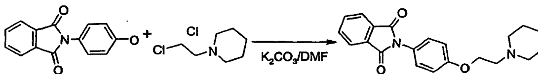
SCHEME VI
