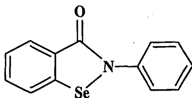
Ebselen
