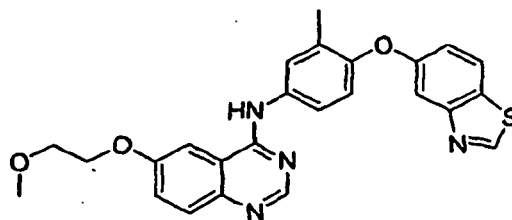
N-(4-benzo[d]thiazol-5-yloxy)-3-methylphenyl)-6-(2-methoxyethoxy)quinazolin-4-amine hydrochloride
