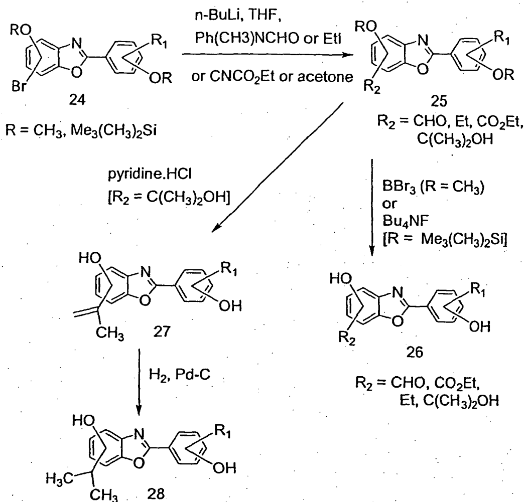
Scheme VI
