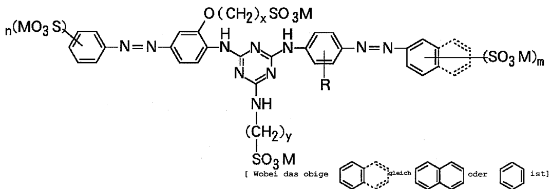
Allgemeine Formel (III)
