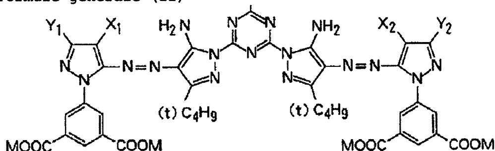
Formule générale (II)
