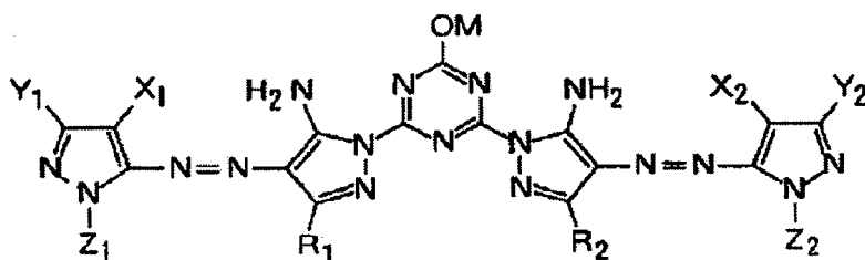
Formule générale (I)
