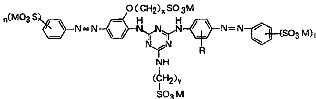
Formule générale (IV)
