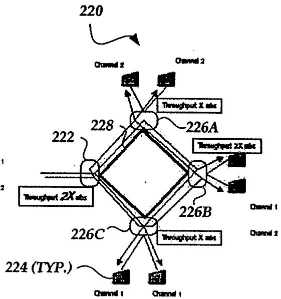
Multicast Enabled DSLAM
