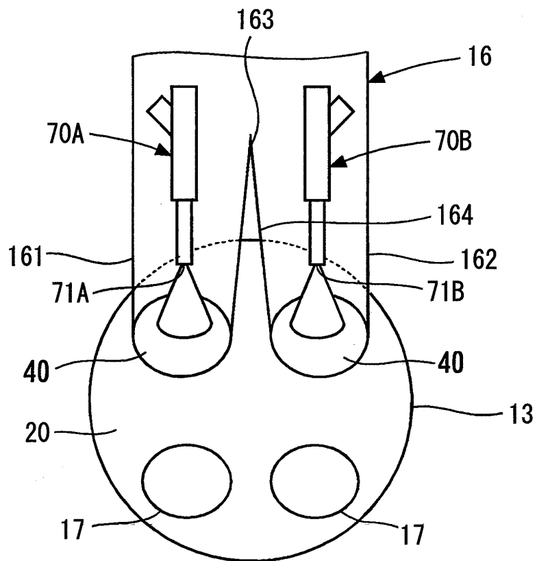
FIG. 25(A)
