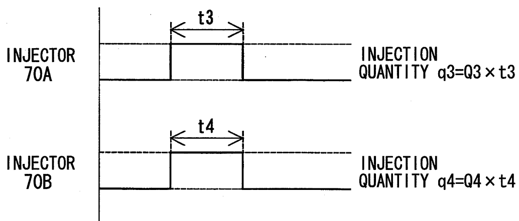
FIG. 25(B)
