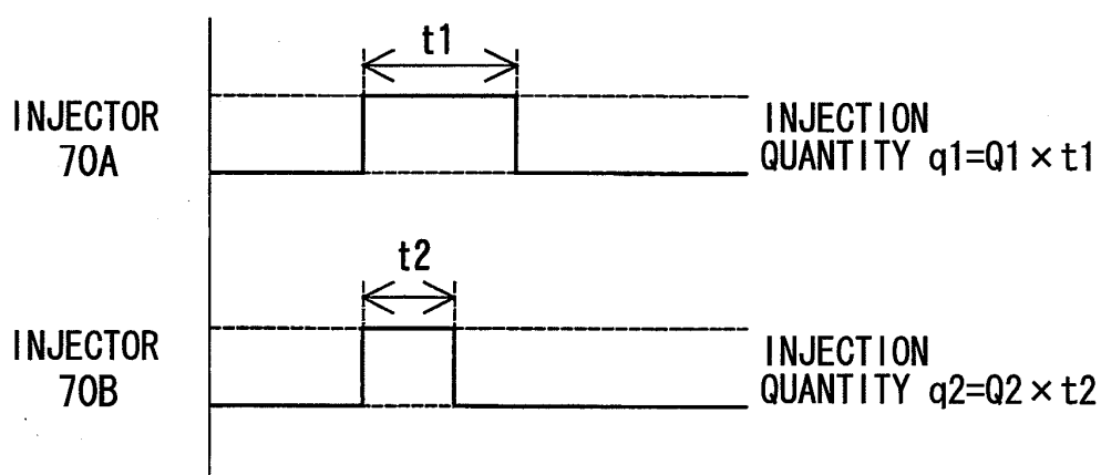
FIG. 22(B)
