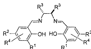
Salen Ligand (28')
