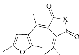
Fulgides (X=O)
