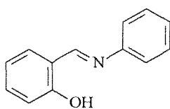
Anil
