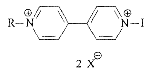
Viologen
