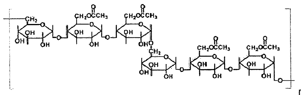
【Chemical Formula 1】
