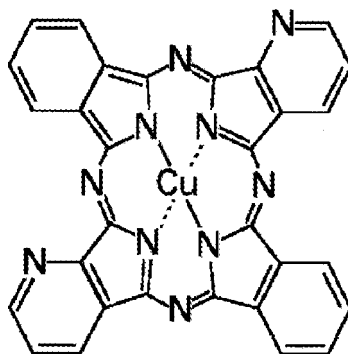
Structural formula 1E
