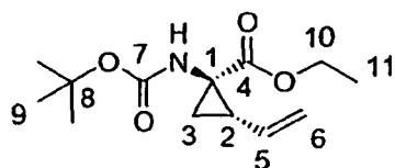
1R, 2S-ester
