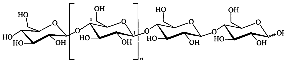
cellulose
