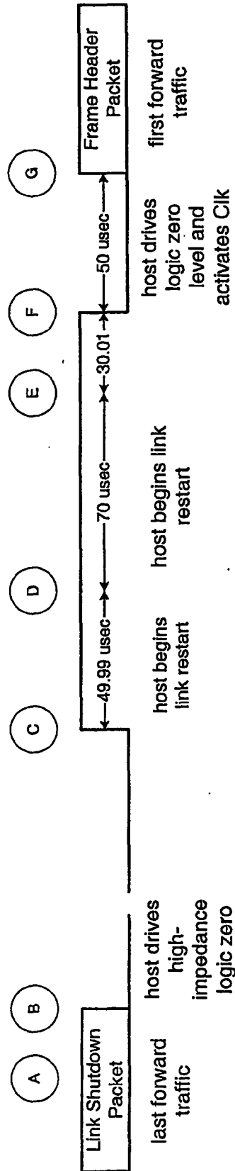
FIG. 39
