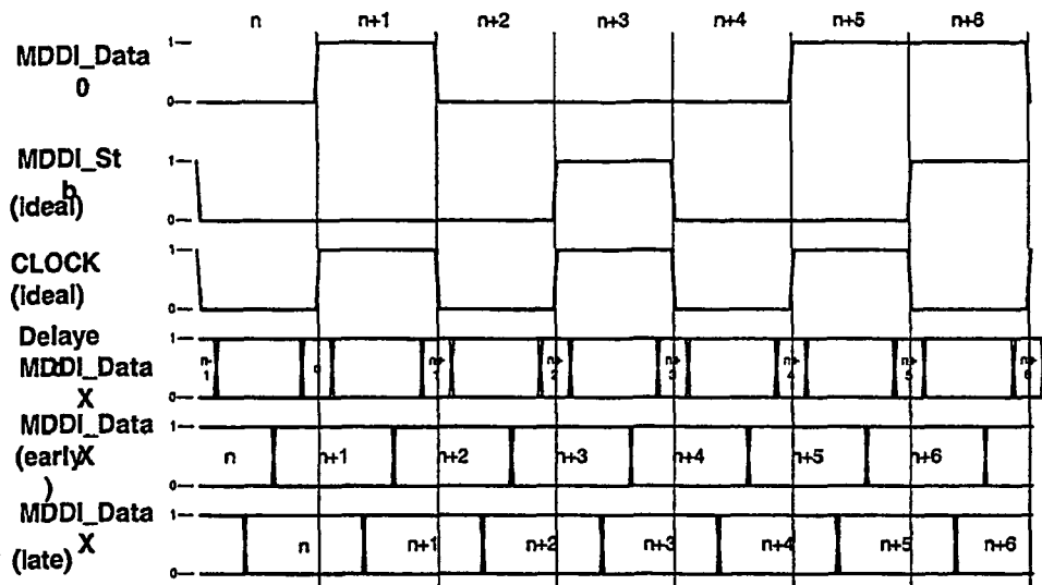
FIG. 60A
