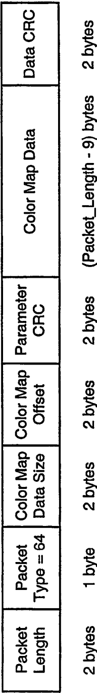
FIG. 16
