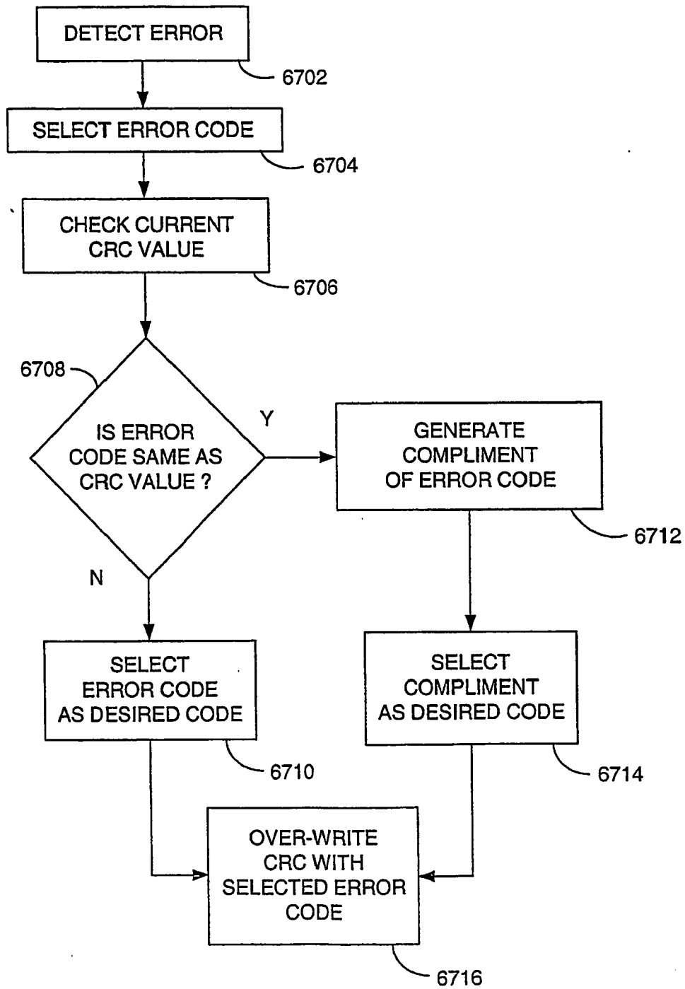
FIG. 67A
