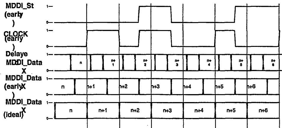
FIG. 60B
