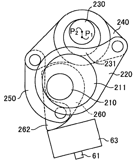
FIG. 8B
