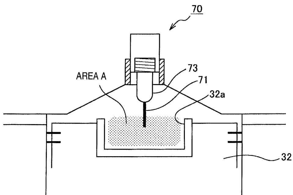
FIG. 23B
