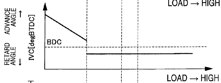
FIG. 10D
