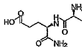
D-Ala-L-isoGln
