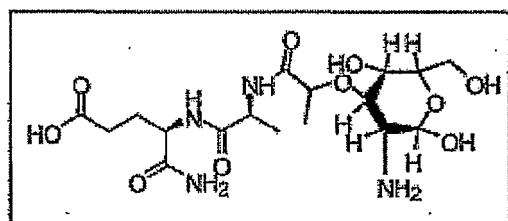
Hyphin (dAcMDP)
