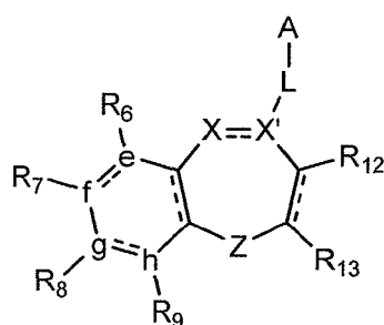
(XV)
