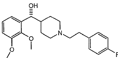
(XIV)
