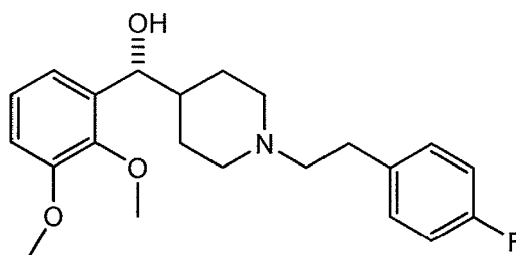
(XIV)
