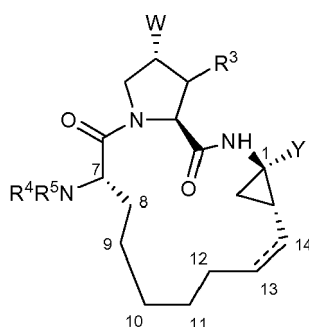
(VIa)
