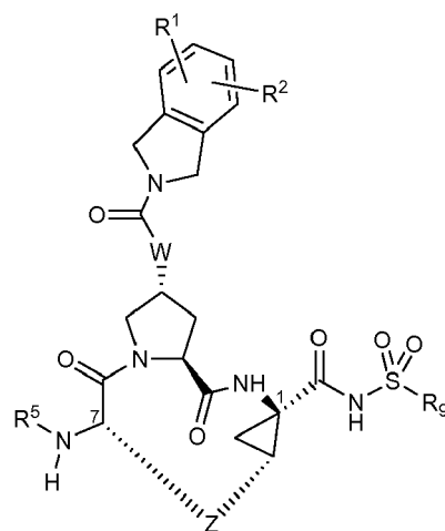
(VIIIb)
