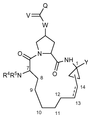
(VII)
