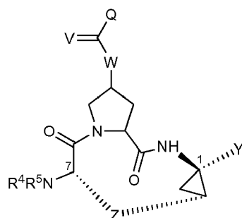
(VIII)
