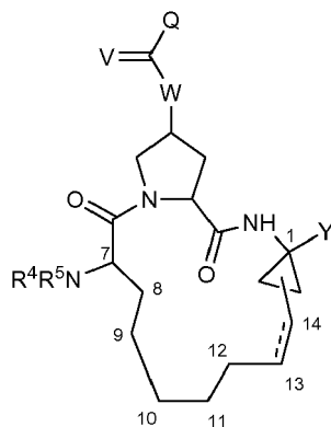
(VII)
