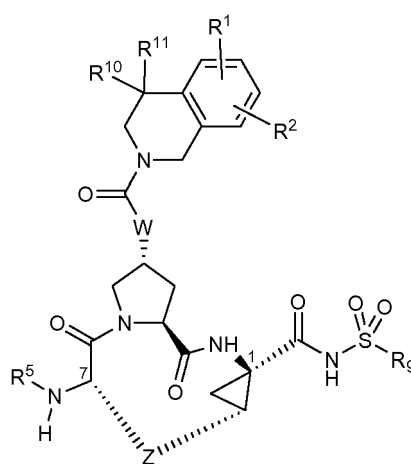
(VIIIa)
