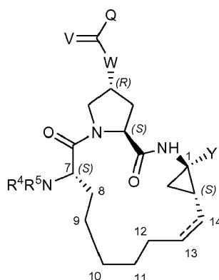
(VIIa)
