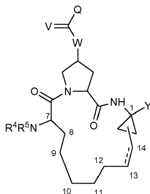
(VII)
