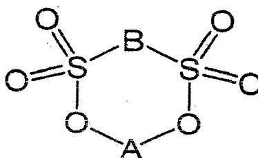
Formule chimique 1
