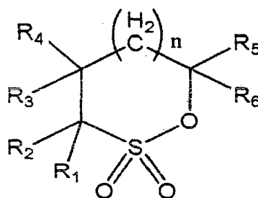
Formule chimique 3
