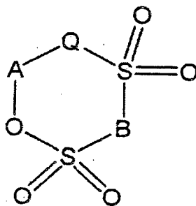
Formule chimique 2
