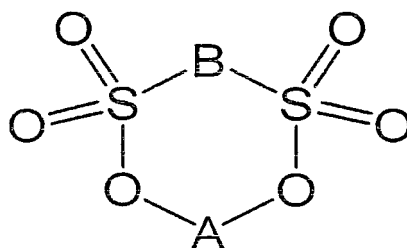
Chemische Formel 1
