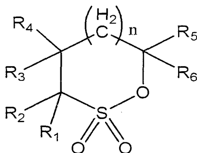
Chemische Formel 3
