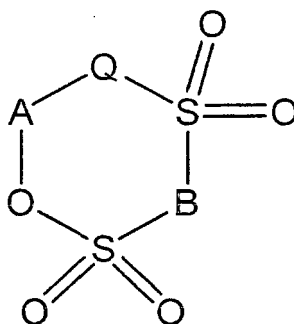
Chemische Formel 2
