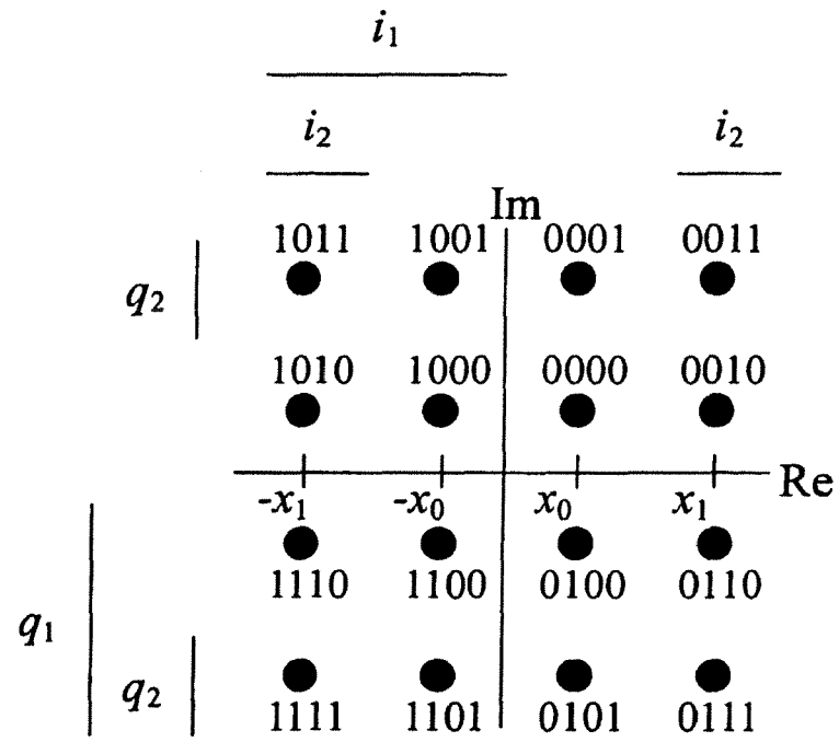
Mapping 1 (bit-mapping order: i_1 q_1 i_2 q_2 )
