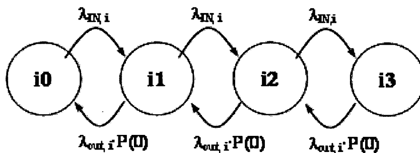
FIG. 10B
