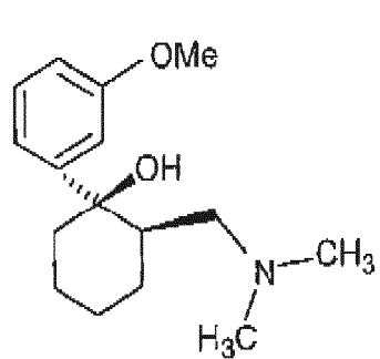
(+) (R,R) cis
