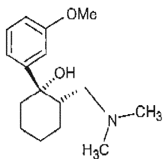
(-) (S,S) cis
