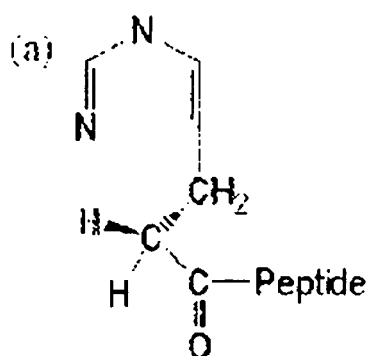
Des-amino-histidyl (DA)-Exendin-4
