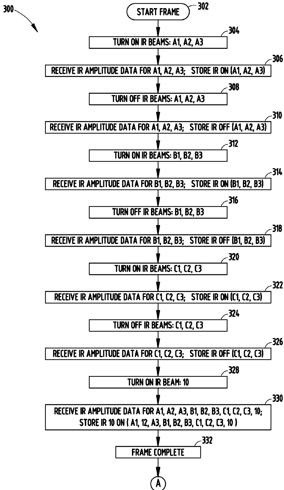
FIG. 18A
