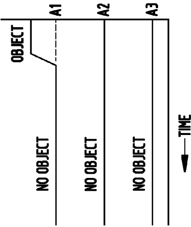
FIG. 15B-B
