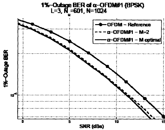
Fig. 5. \alpha -OFDM#1 BER
