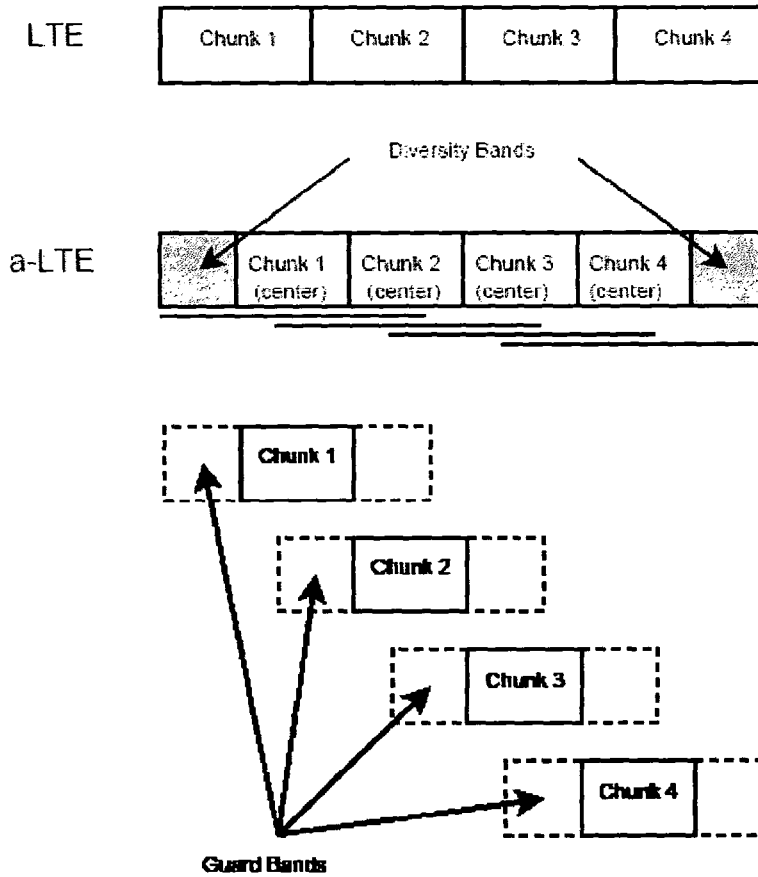
Fig. 8. \alpha -LTE
