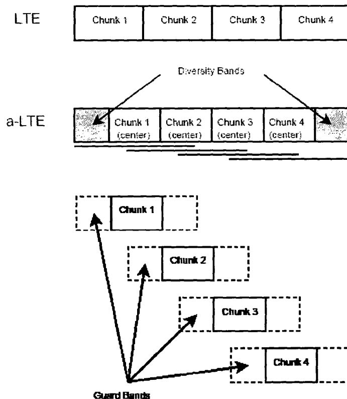
Fig. 8. \alpha -LTE
