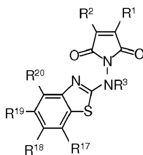
( VII )
