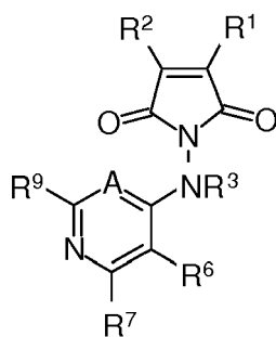
( XI )
