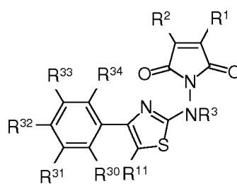
( X )
