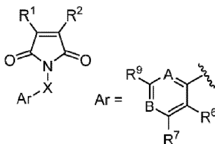
Struktur (II)
