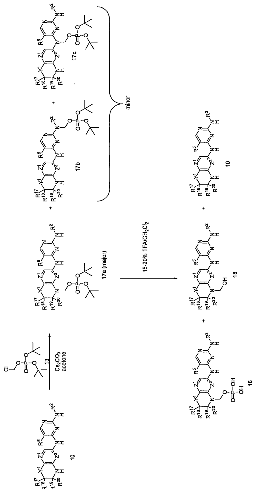
Scheme (IV)
