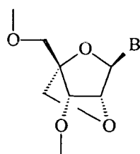
2'-4' D-form LNA 1'R, 3'S, 4'R
