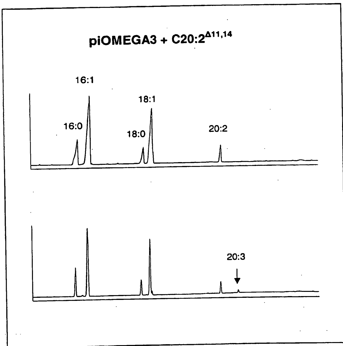
Figur 14: Desaturierung von C20:2 \omega -6-Fettsäure zu C20:3 \omega -3-Fettsäure durch Pi-omega3Des.
