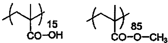
Binder polymer (1)
