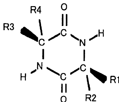
Allgemeine Strukturformel (1),
