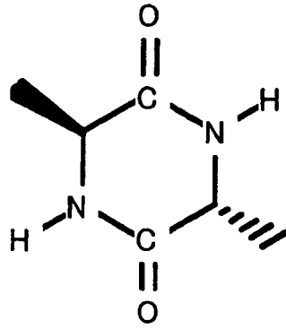
Anhydride DL-Alanine
