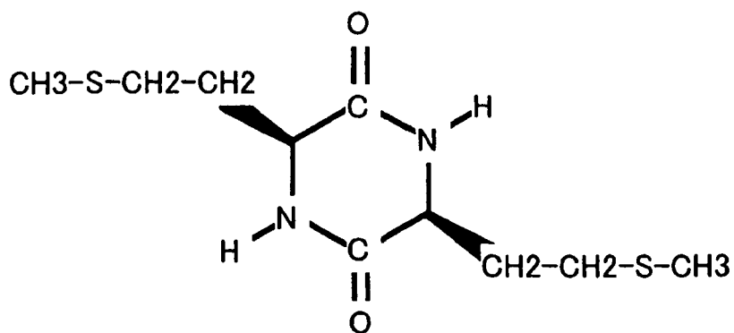
Anhydride L-Methionine
