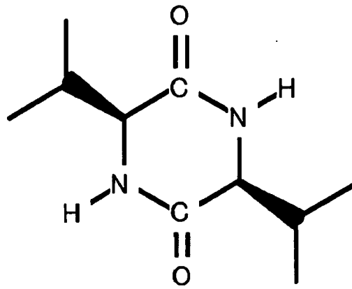
Anhydride L-Valine
