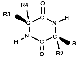
formule de structure générale (1)
