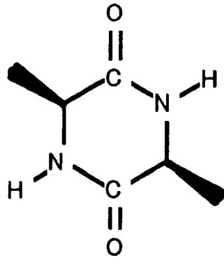
Anhydride L-Alanine
