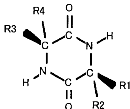
Allgemeine Strukturformel (1),
