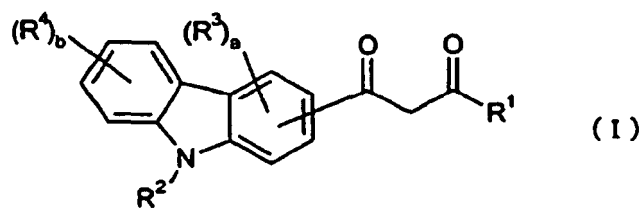
[Formule 1]
