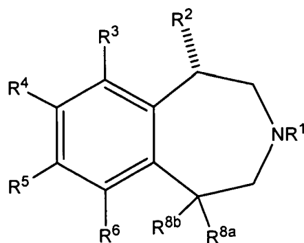
Va
