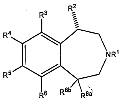
Va
