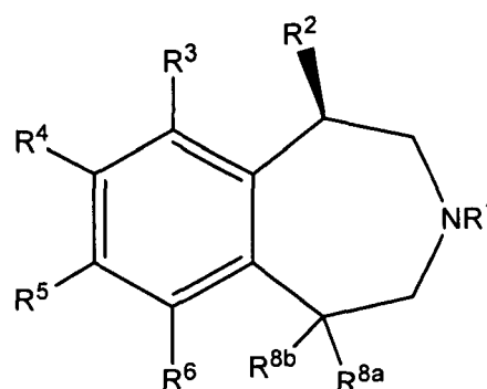
Vb
