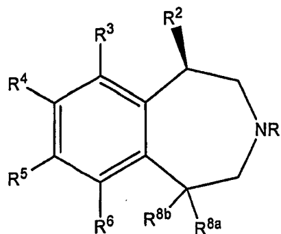
Vb
