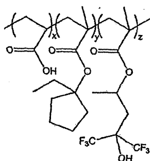
xyxxxyy/zzzzzz di-block
