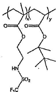
xxxx/yyyyy di-block
