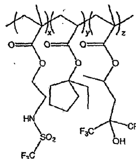
xxxx/zyzzzyzy di-block
