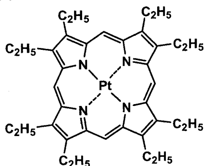
Pt-3
