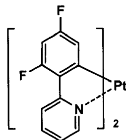
Pt-2
