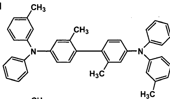
HMTPD
