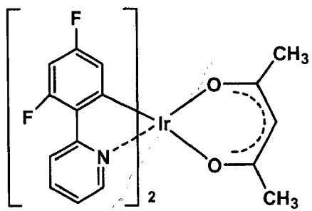
Ir-10
