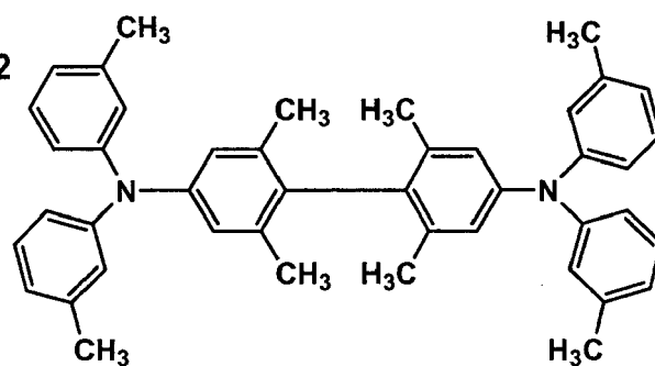
m-MTDATXA
