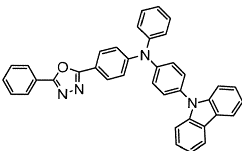
YGAO11
