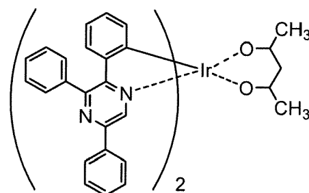
Ir(tppr) 2 acac
