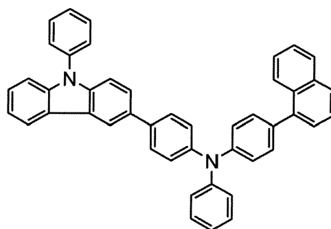
PCBANB
