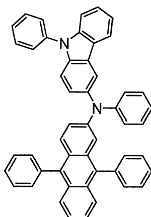
2PCAPA
