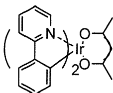
Ir(ppr) 2 acac
