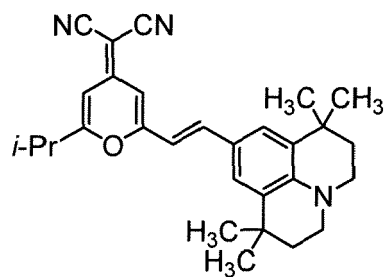
DCJTl
