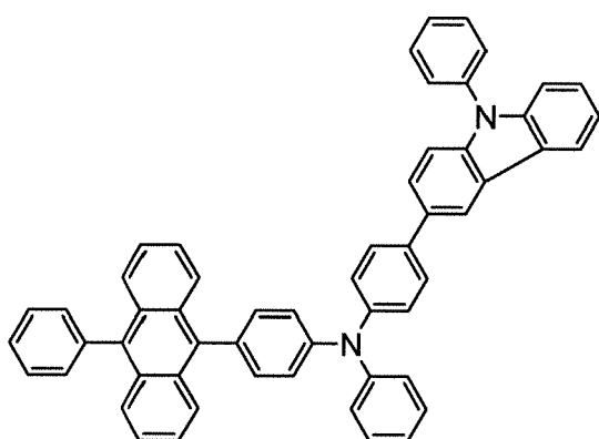
PCBAPA
