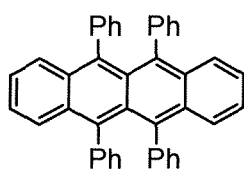
Rubrene
