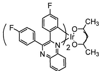
Ir(Fdpq) 2 (acac)
