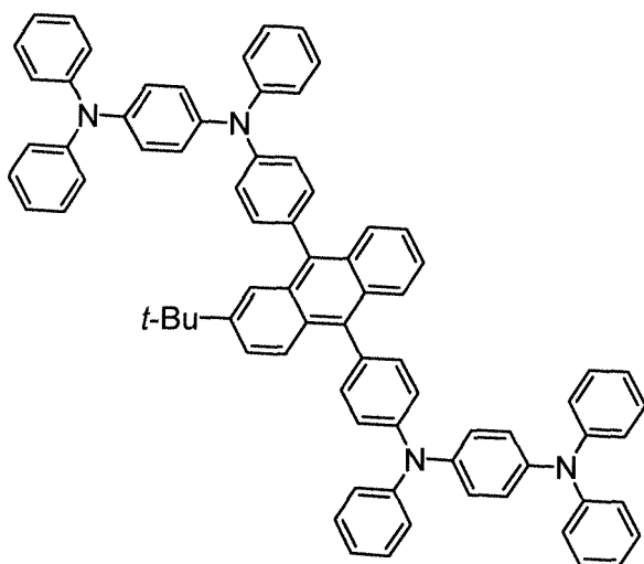
DPABPA
