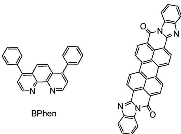
PTCBI
