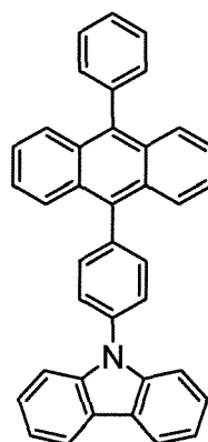
CzPA
