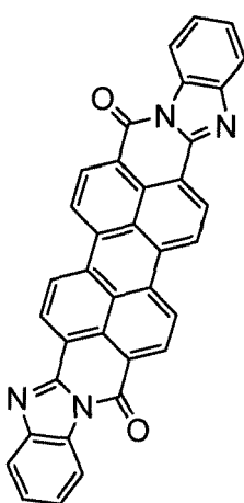
PTCBI
