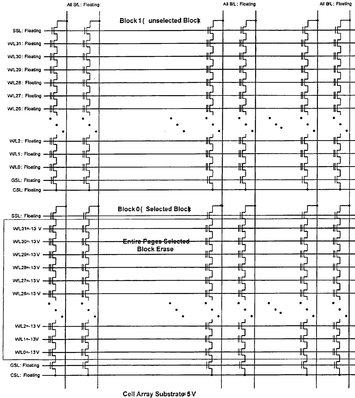
Fig. 27
