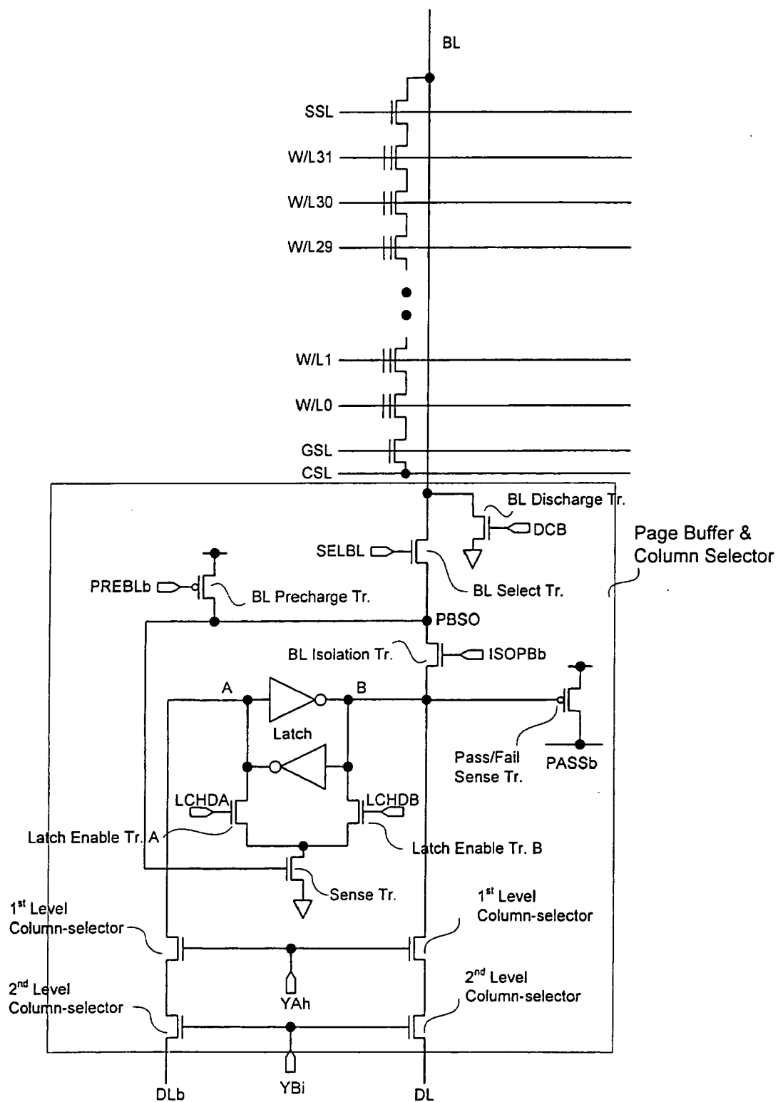
Fig. 36
