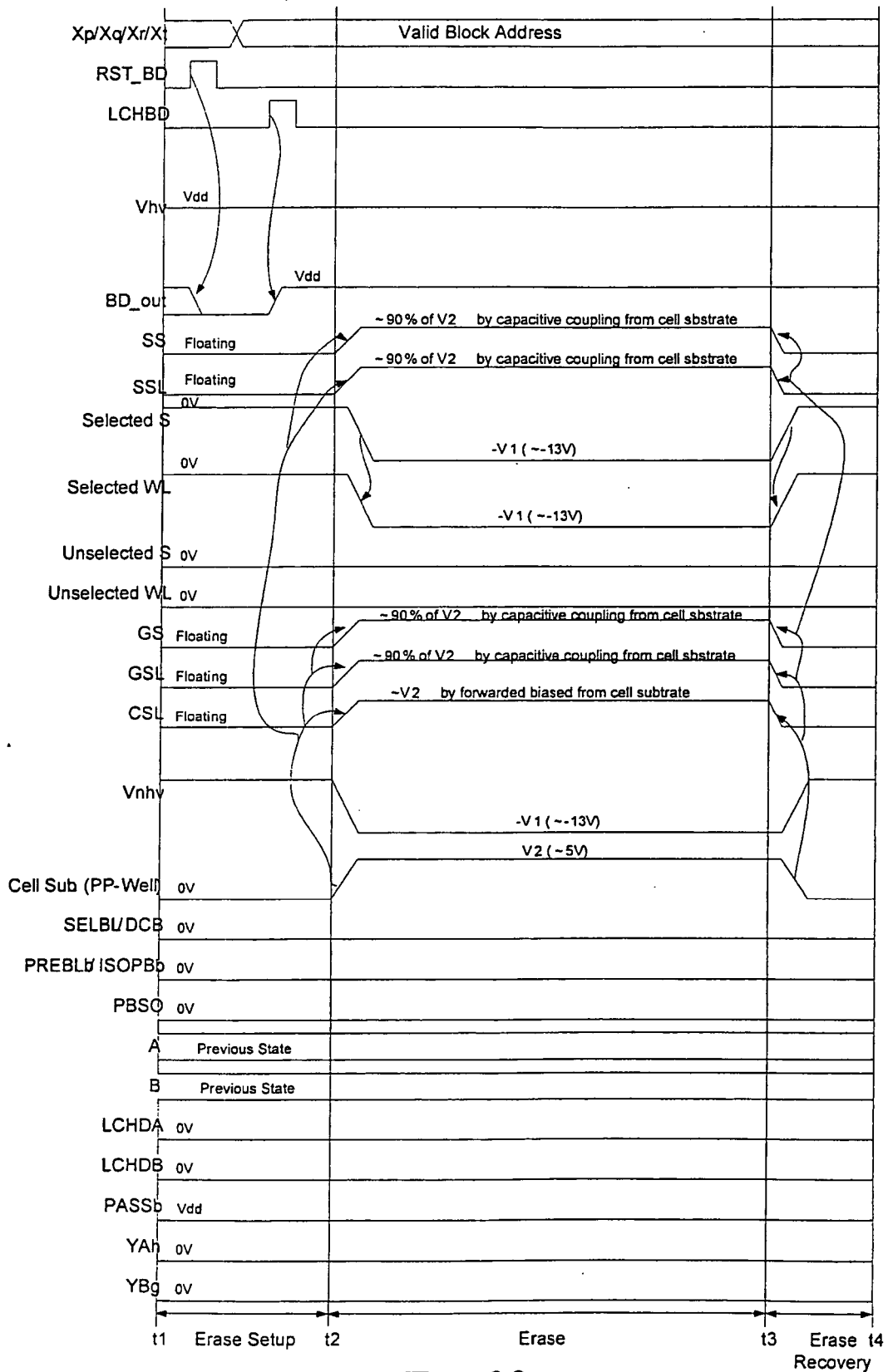
Fig. 39
