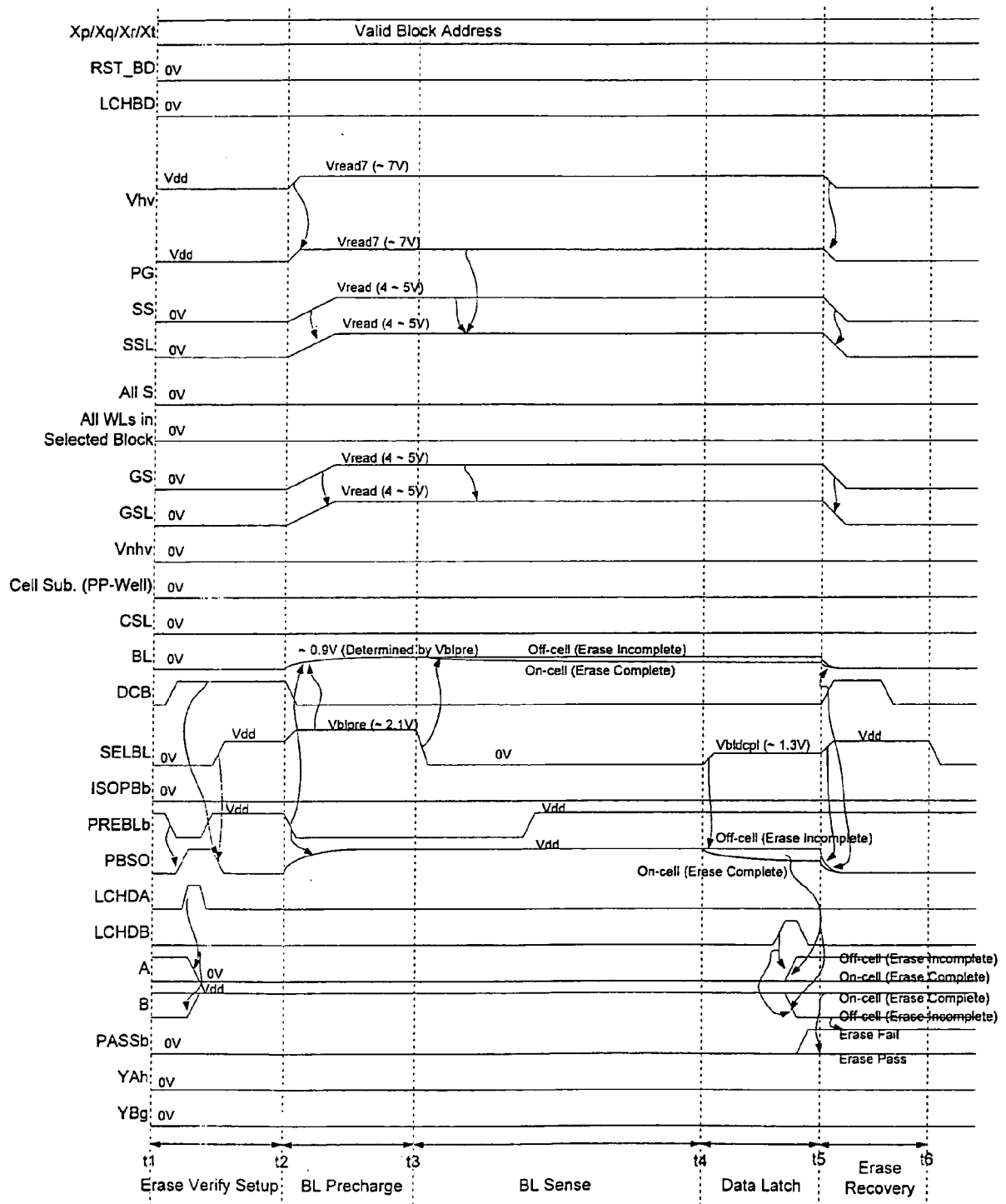
Fig. 45
