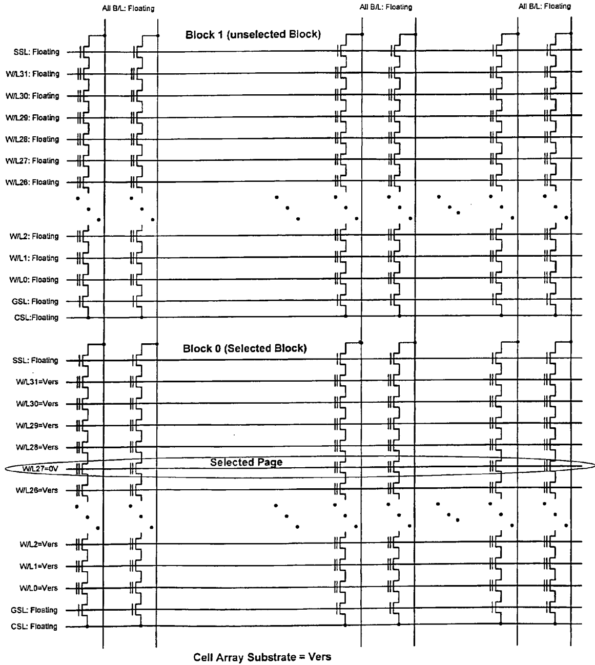
Fig. 18
