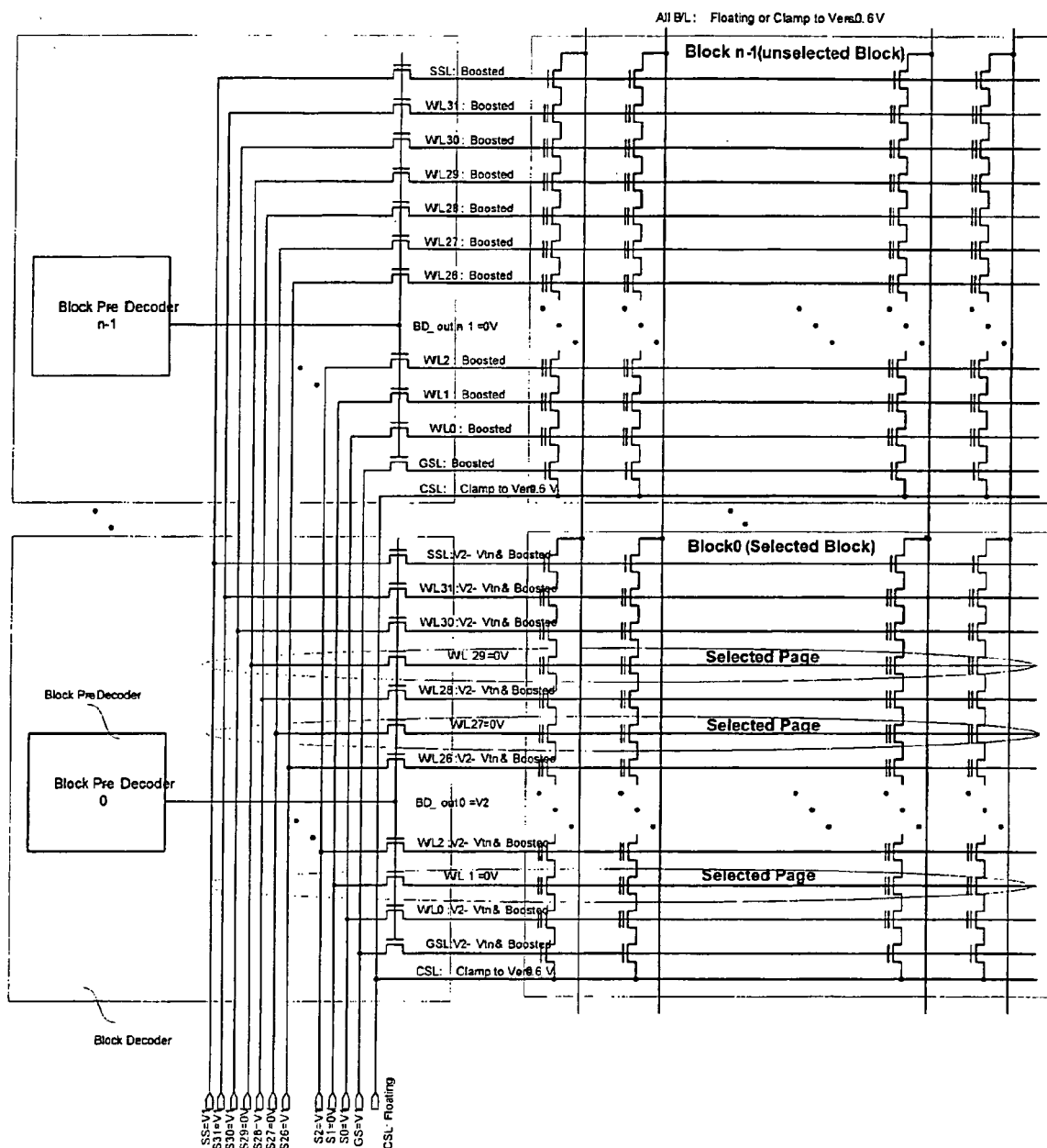
Fig. 49
