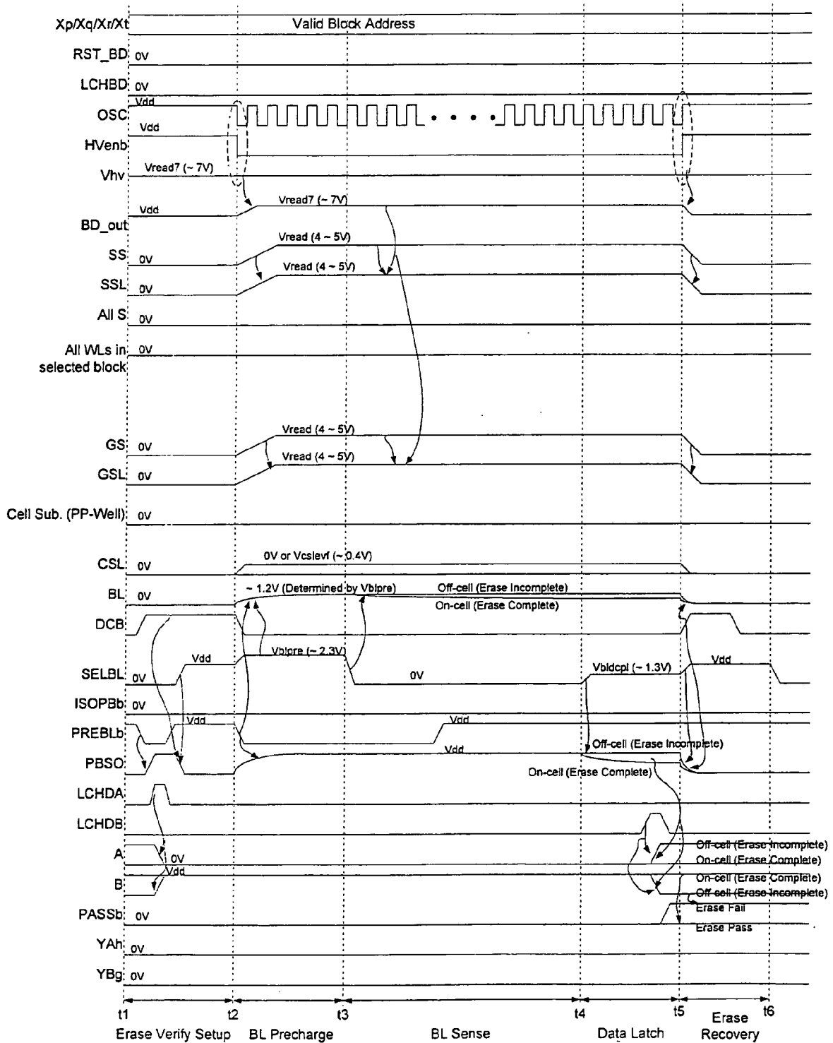
Fig. 43
