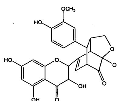
silidianin
