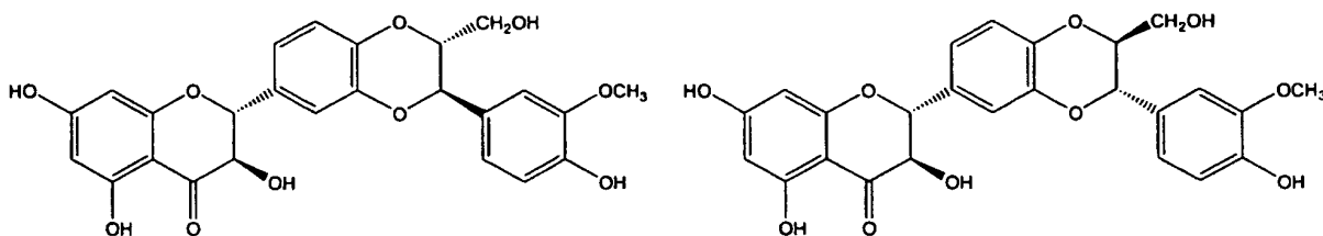
silibinin A
