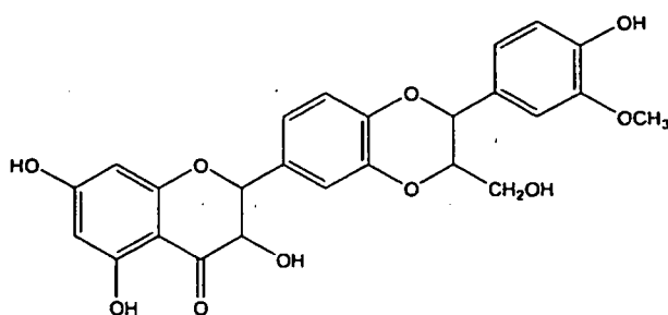
isosilibinin
