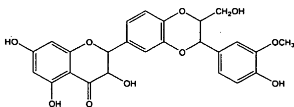
silibinin
