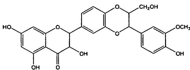
silibinin
