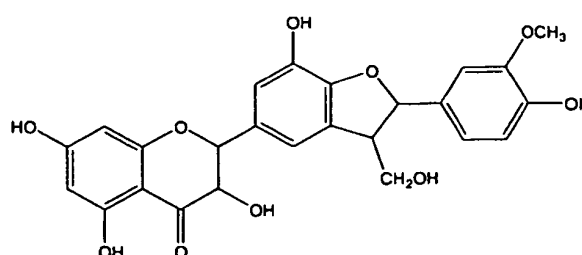
silichristin
