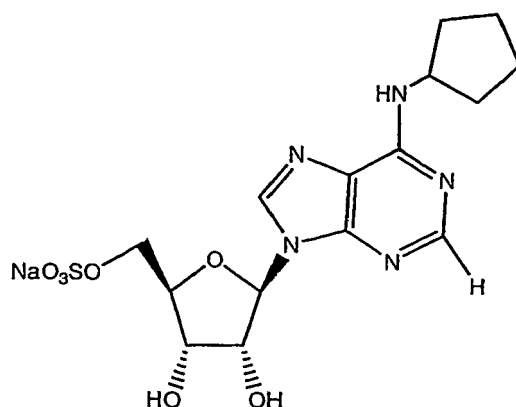
23 (sodium salt)
