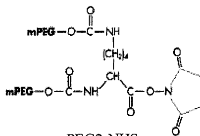
mPEG2-NHS
