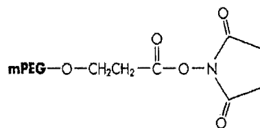
mPEG-SPA
