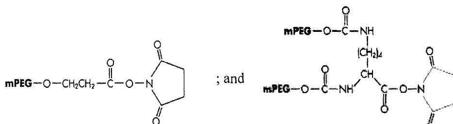
mPEG2-NHS
