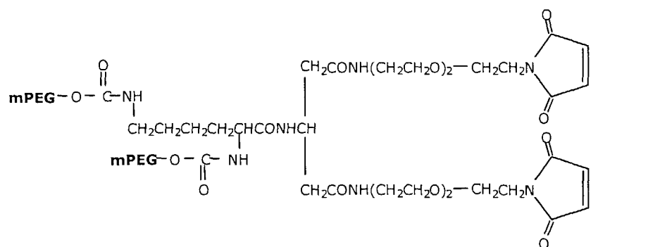
mPEG2-(MAL) 2
