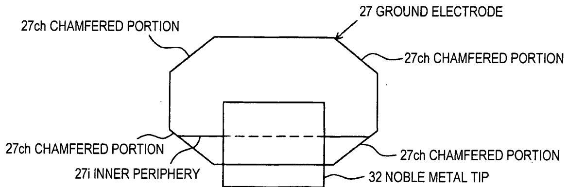
FIG. 14C
