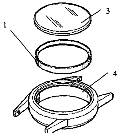
Fig. 1.2 (art antérieur)
