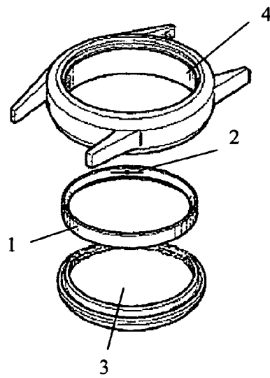
Fig. 6.2
