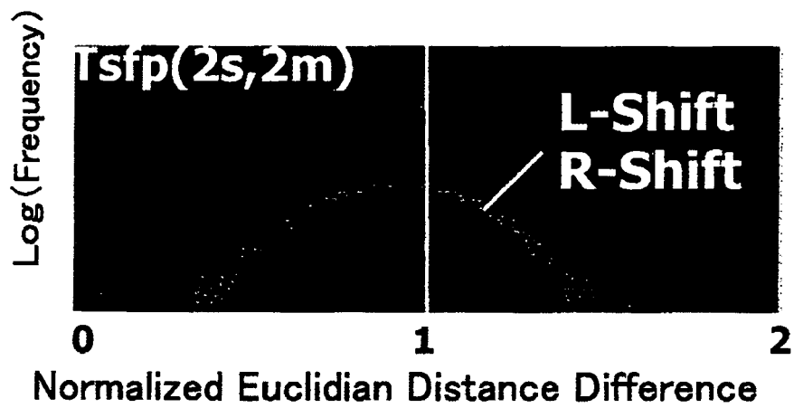
(a) Tsfp(2s,2m) Edge Shift = 0.0T
