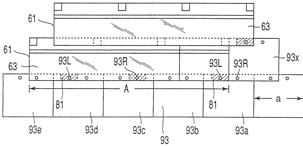
FIG. 24B
