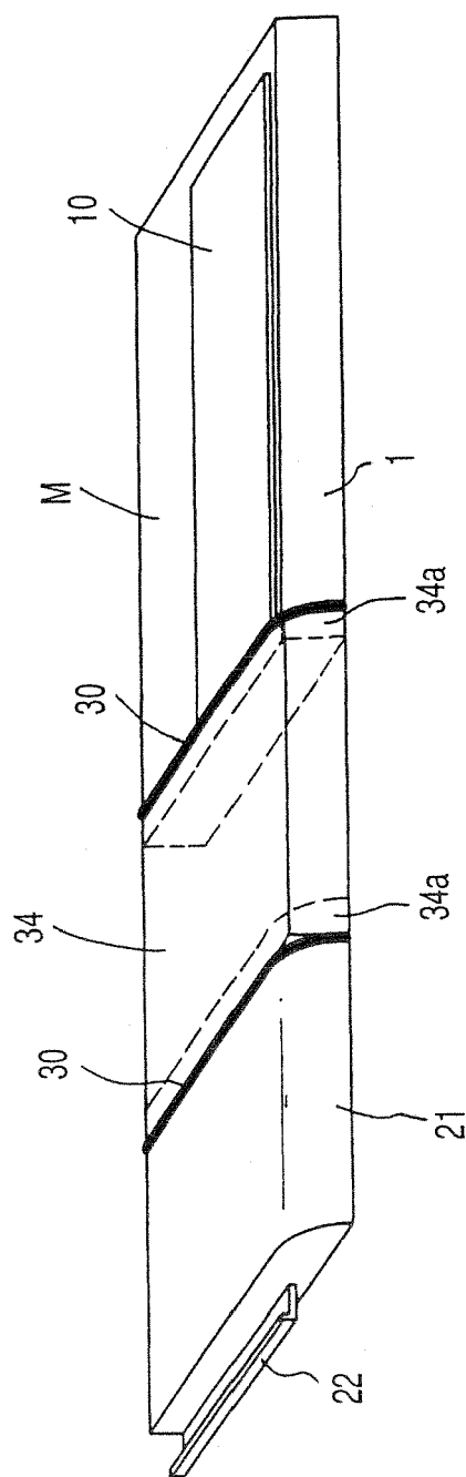
FIG. 13
