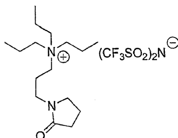
Cyclic amide IL 2
