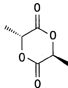
RS or meso-lactide
