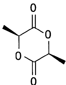
SS or L-lactide
